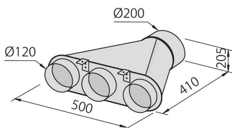
Collettore per 3 tubi 2524 000
